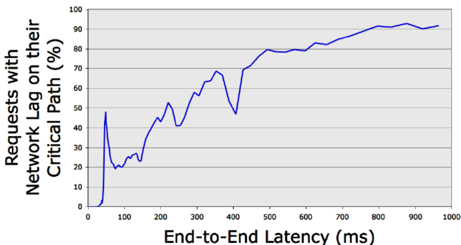
图7：全局搜索的跟踪片段，在不常遇到高网络延迟的情况下，在沿着关键路径的端到端的请求延迟，如图所示。
